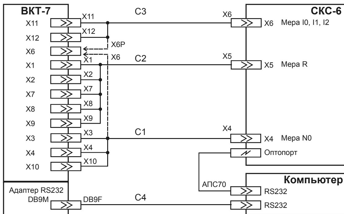
Рисунок 8.1 – Схема поверки
